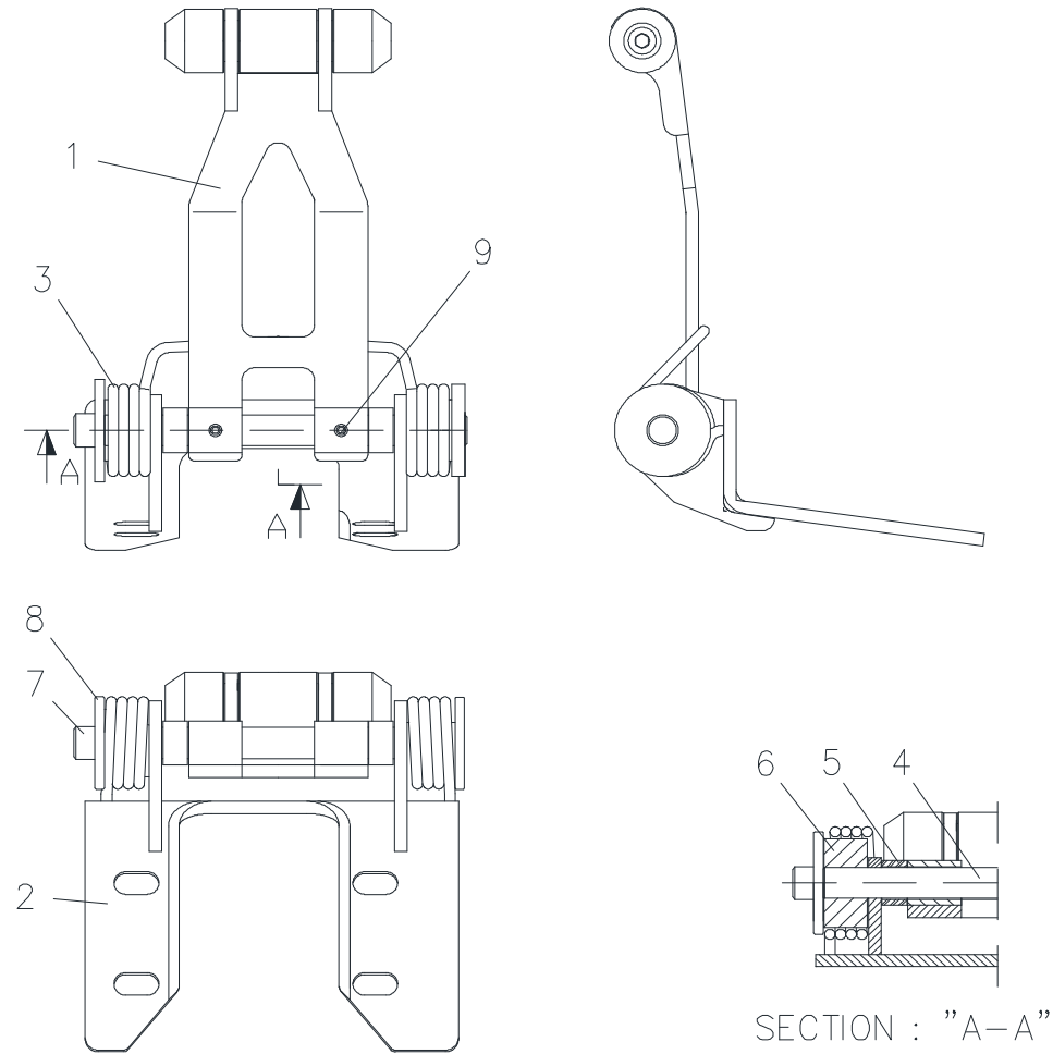
Fig. 2-2-3 SAC-2501R WIRE GUIDE ROLLER
