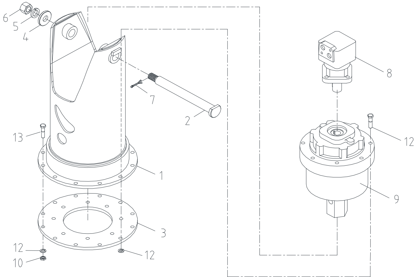
Fig. 5-1 SAC-2501R AUGER MOTOR ASS'Y
