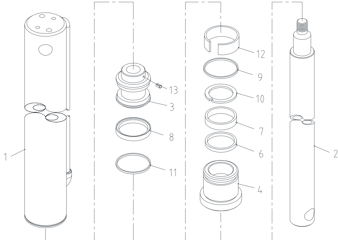
Fig. 3-1 SAC-2501R JACK CYL' ASS'Y
