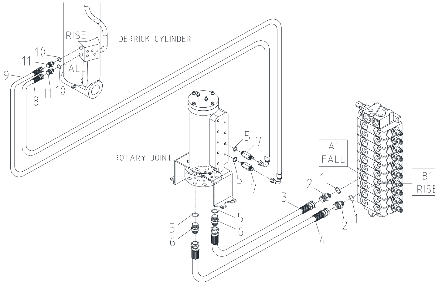
Fig. 4-2 SAC-2501R DERRICK PIPING
